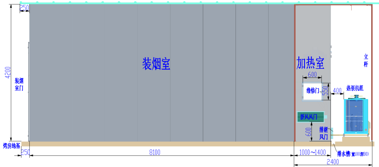
图 1 烤房左侧视图
