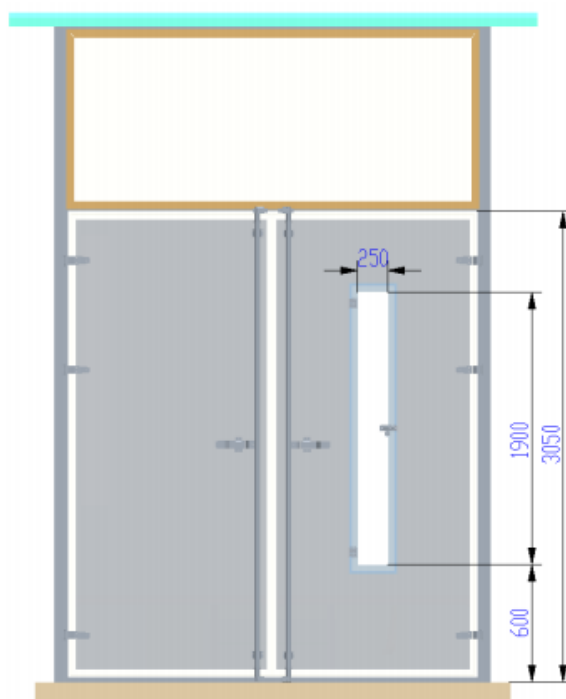
图 8 装烟室大门
