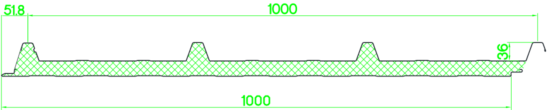
图 5 屋顶板视图
