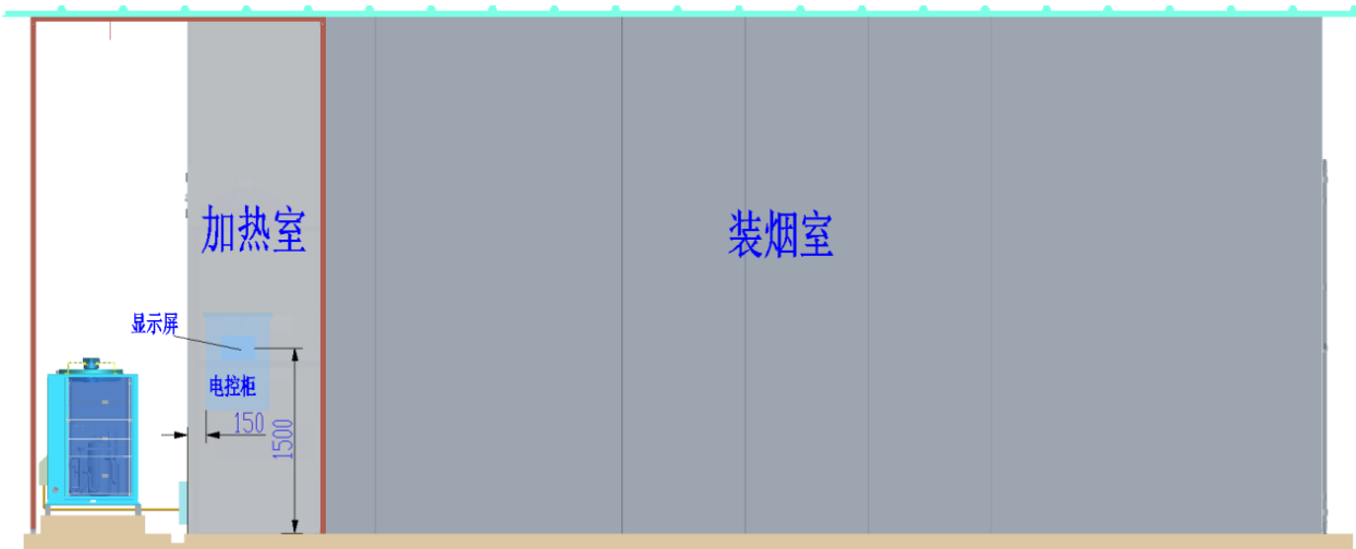
图 2 烤房右侧视图
